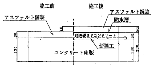
図3 床版補強（増厚）断面
