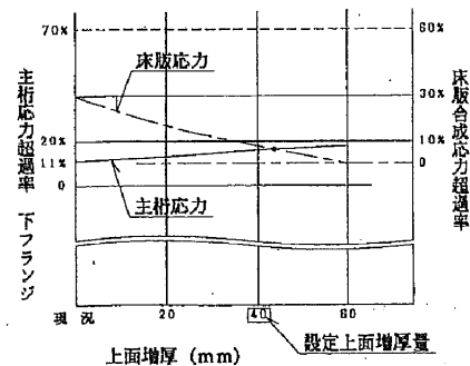
図2 コンクリート増厚—発生応力関係図
