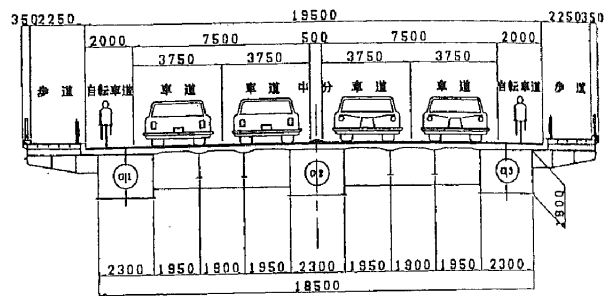
図1 橋梁標準断面図
