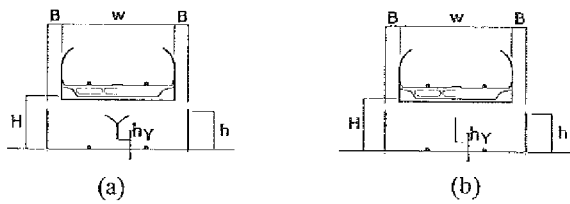
図-4 吸音板空隙高さに対する騒音低減効果
